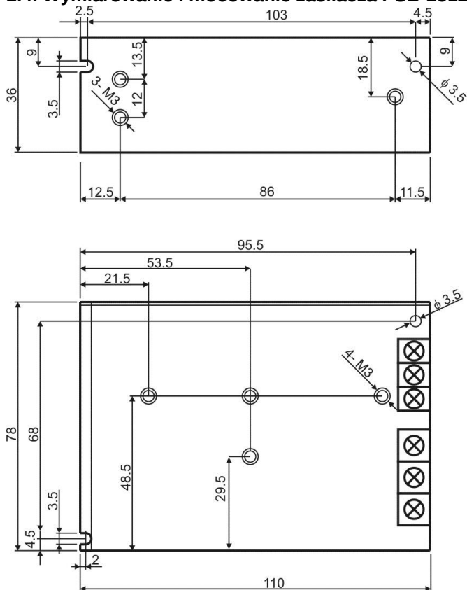
Rysunek 2. Widok mechaniczny zasilacza.
